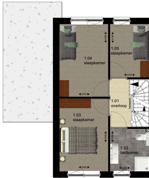
Verdieping
