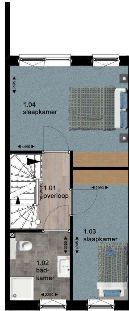
Verdieping
